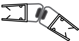
Magnetdichtung 135° Paarweise 900102
